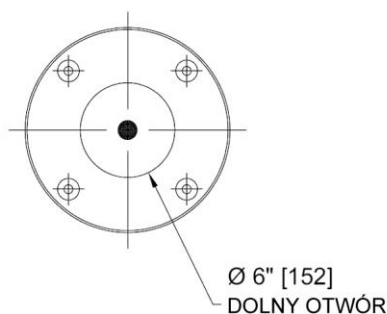
WIDOK PODSTAWY
